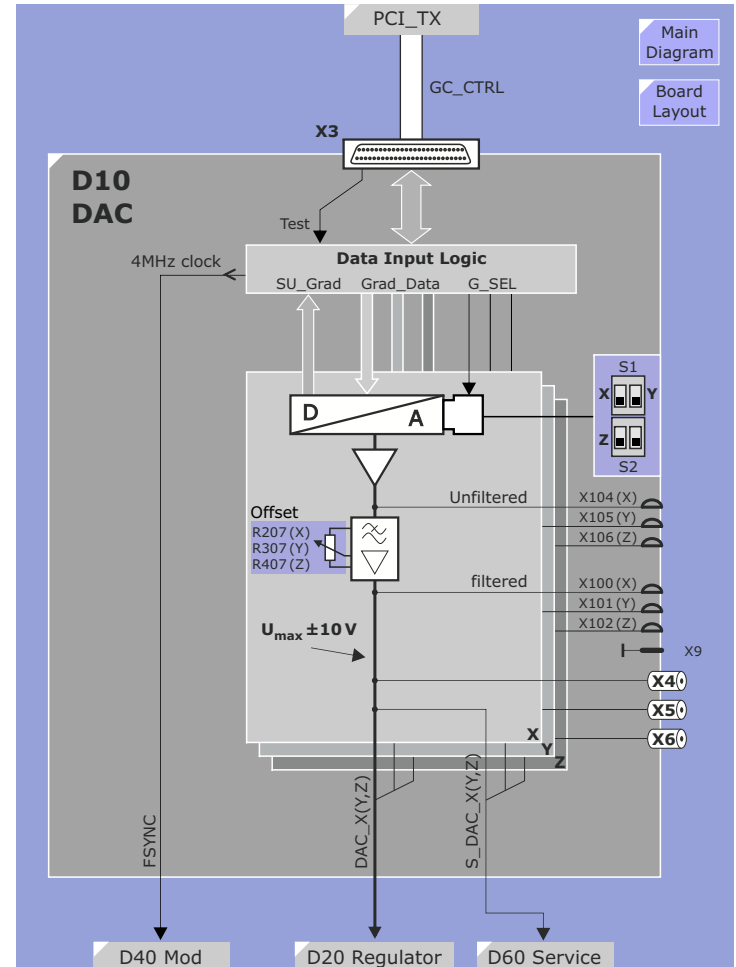
Figure 127 D10 DAC
