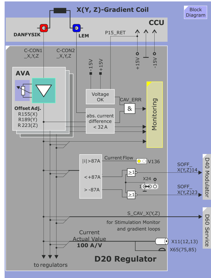
Figure 132 D20 Actual Value Amplifier
